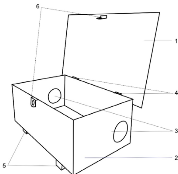
Рисунок 1. 1 – крышка; 2 – корпус; 3 – входные отверстия; 4 – шарнирные петли; 5 – ножки; 6 – проушины
